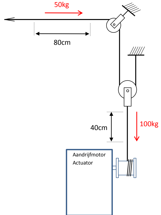
Uitscharen Movable pulley system
